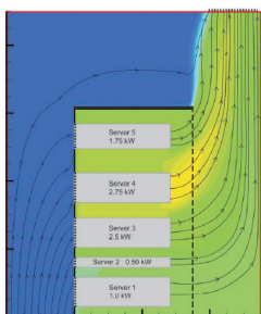
Nachher: Durch die 99,95% Abdichtung mit HotLok kommt es zu einer optimalen Nutzung der vorhandenen Kühlungskapazität.
