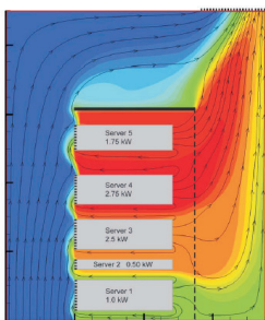
Vorher: Hotspots (rot) im 19" Rack
